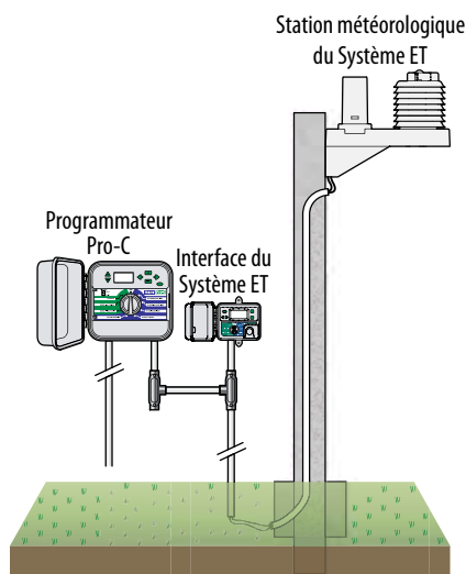
La Sonde ET peut être montée sur un mur ou sur un poteau jusqu'à 30 mètres de distance du module ET.
