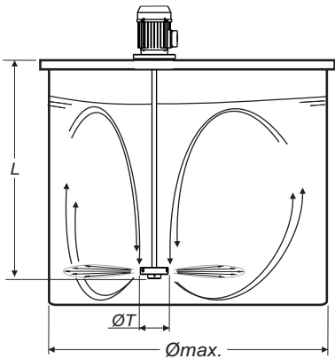
DIMENSIONES / DIMENSIONS
